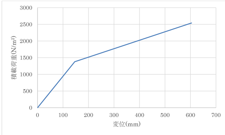
グラフ 3 荷重・変位関係 (試験体 No.3)
