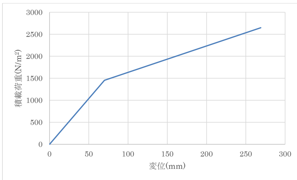
グラフ 1 荷重・変位関係 (試験体 No.1)
