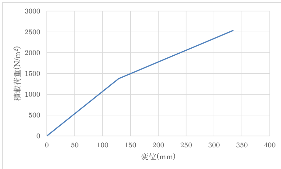
グラフ 4 荷重・変位関係 (試験体 No.4)
