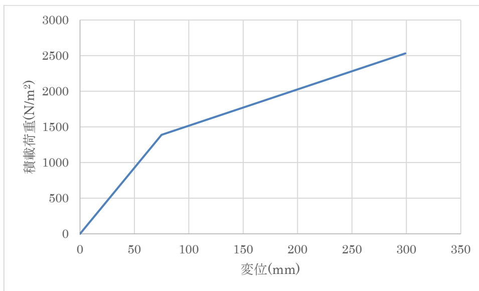
グラフ 2 荷重・変位関係 (試験体 No.2)
