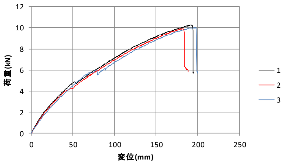
図 3 荷重-変位関係 (シリーズ No.1)
