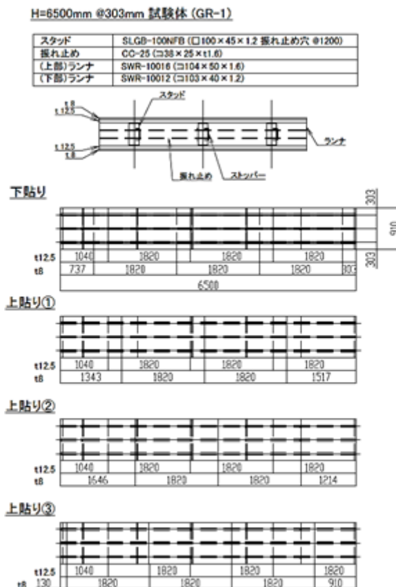
図 1 試験体図面 (シリーズ No.1)
