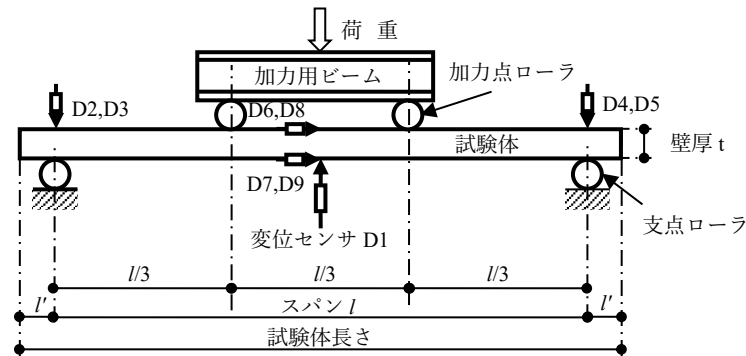
図 1 载荷試験方法
