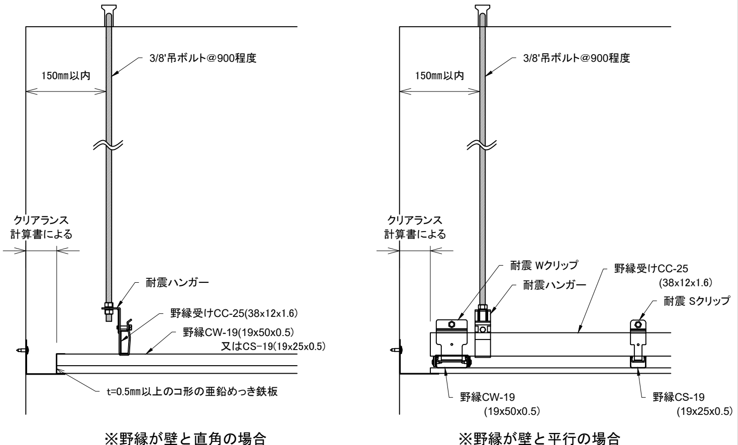
[図2：野縁及び野縁受け端部の納まり]
