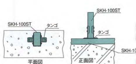
▼ (3) タンゴ (PAT.)
