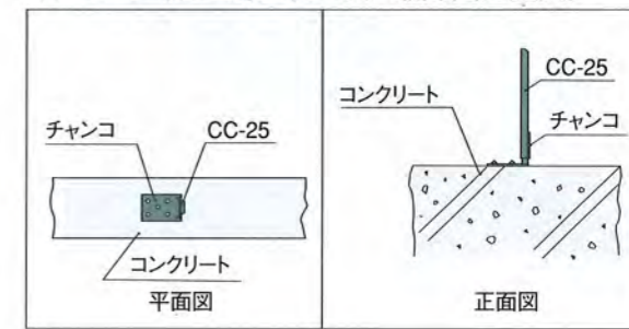
4. ◆ チャンコ (チャンネル端部固定金具)
