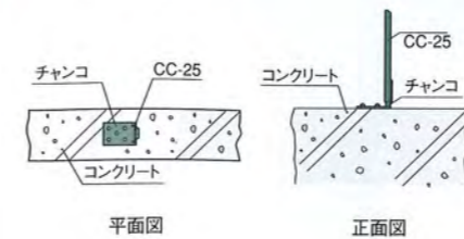
◆ (4) チャンコ
