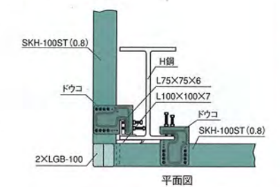
● (6) 出隅部
