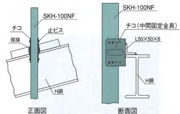
2. ● チコ（中間固定金具）PAT.
