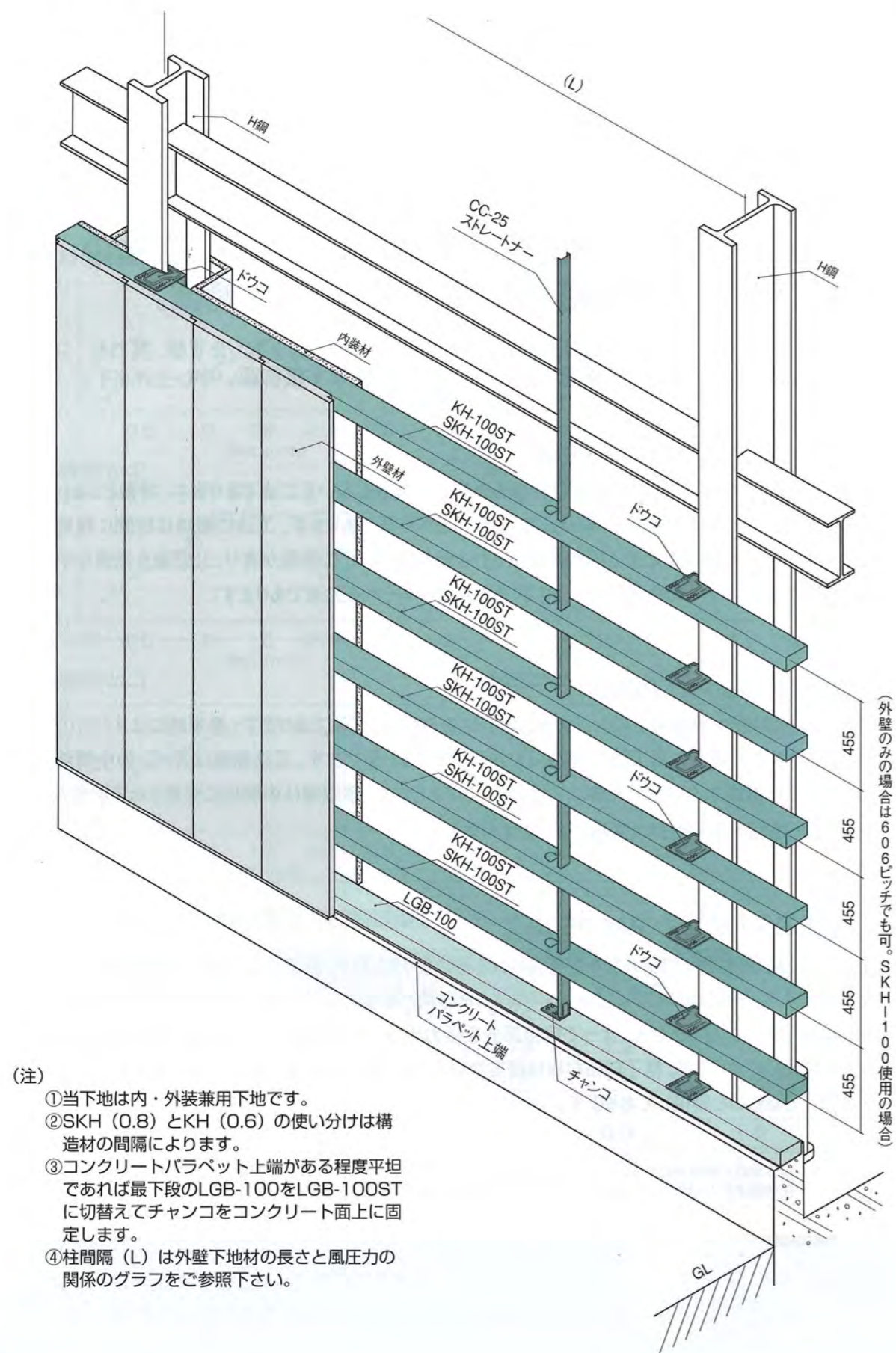
(1) 施工例1
