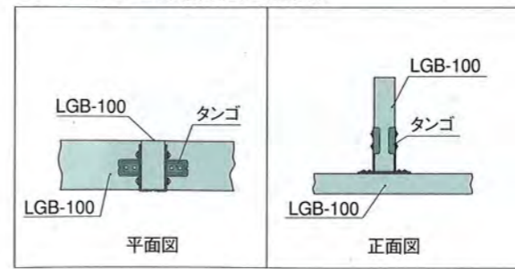
3. ▼ タンゴ (端部固定金具)
