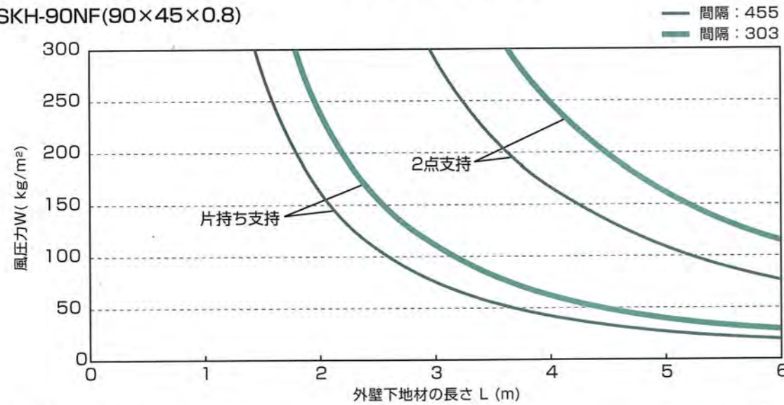
●KH-90NF(90×45×0.6)
