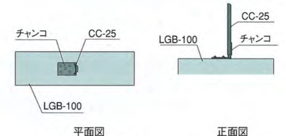
4. ◆ チャンコ（チャンネル端部固定金具）
