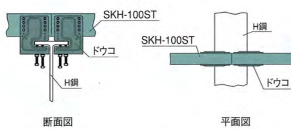
■ (2) ドウコ (胴縁ジョイント部)
