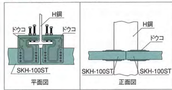
2. ■ 胴縁ジョイント部 (ドウコ)
