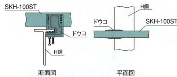
■ (1) ドウコ (胴縁固定金具) PAT.
