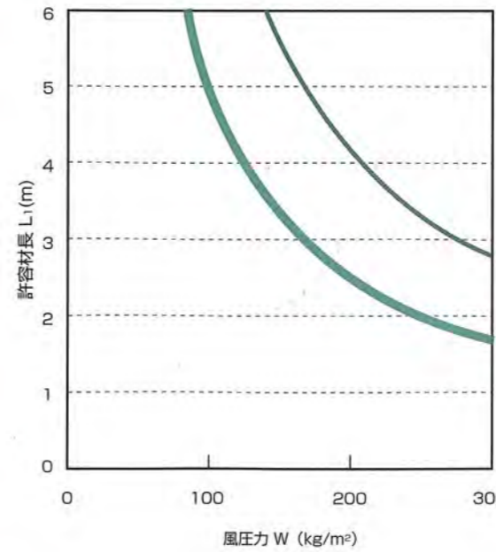
● L_2=3.5\text{m}
