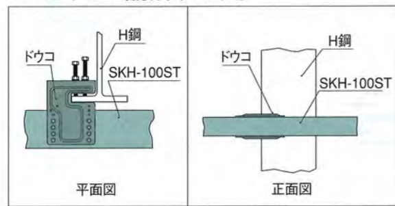
1. ■ ドウコ (胴縁固定金具)
