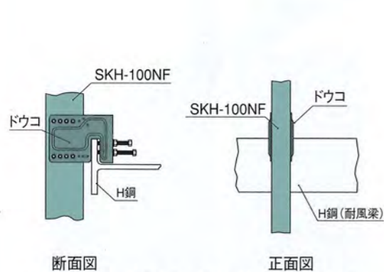
1. ■ ドウコ（胴縁固定金具）PAT.
