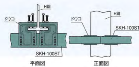
■ (2) ドウコ (胴縁ジョイント部)
