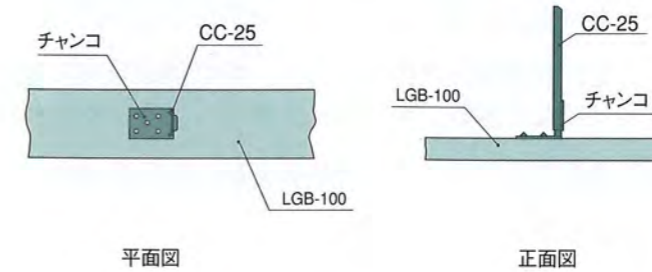
◆ (3) チャンコ (チャンネル端部固定金具)
