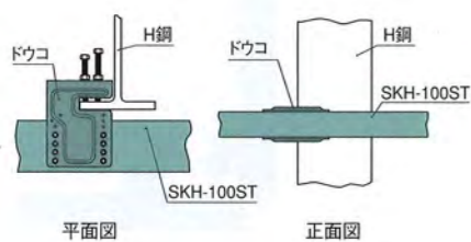
■ (1) ドウコ (PAT.)
