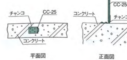
◆ (4) チャンコ
